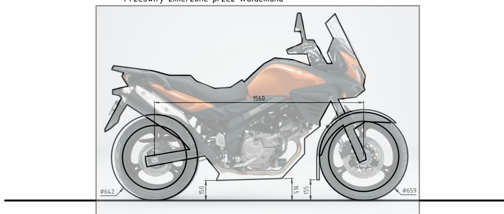
V-Strom 650 - w stanie spoczynku. Przeświły zmierzone przez Waldemana
